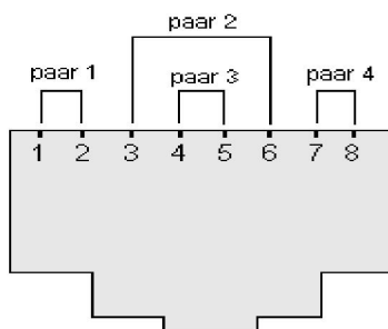
Aansluitingen RJ45 achteraanzicht
